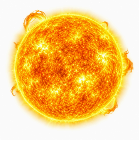
Sonne
