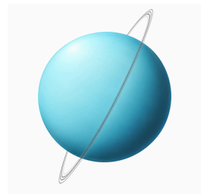
Uranus
